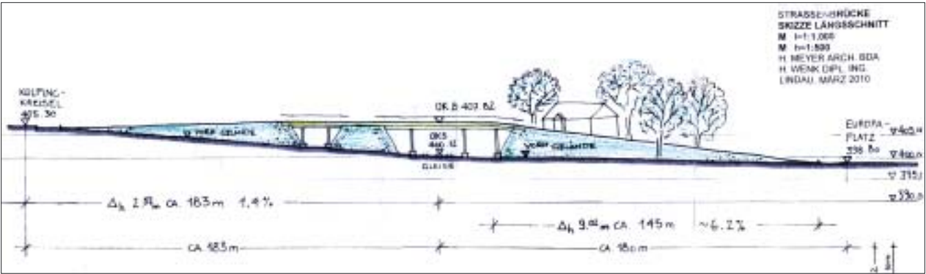
Eine Brücke vom geplanten Kreisverkehr „Kolping-Kreisel“ über die Bahn zum Europaplatz vor der Inselbrücke könnte laut Berechnung der Bürgerinitiative mit einer maximalen Steigung von etwa 6,2 Prozent auf der Südseite auskommen. Planskizze: Meyer/Wenk
