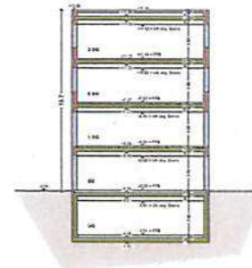
Schnitt 1-1. M 1:200
