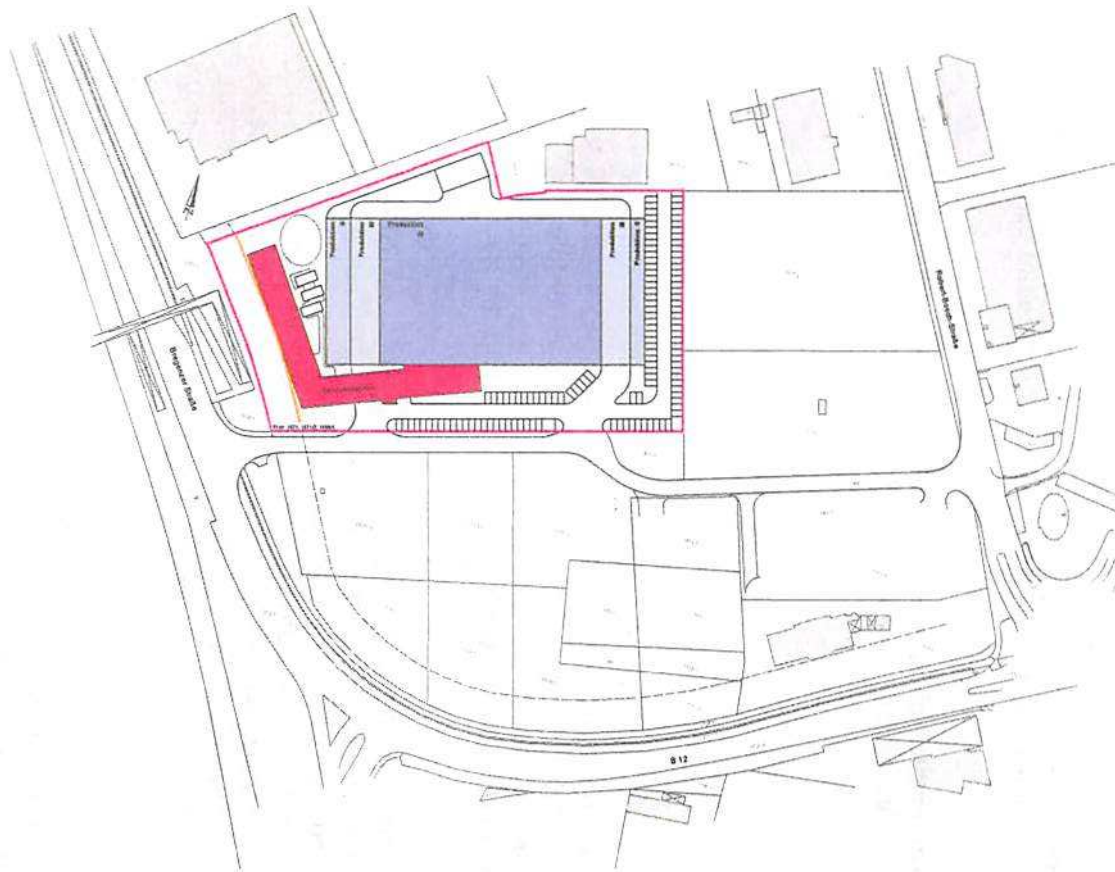
Lageplan. M 1:1000
