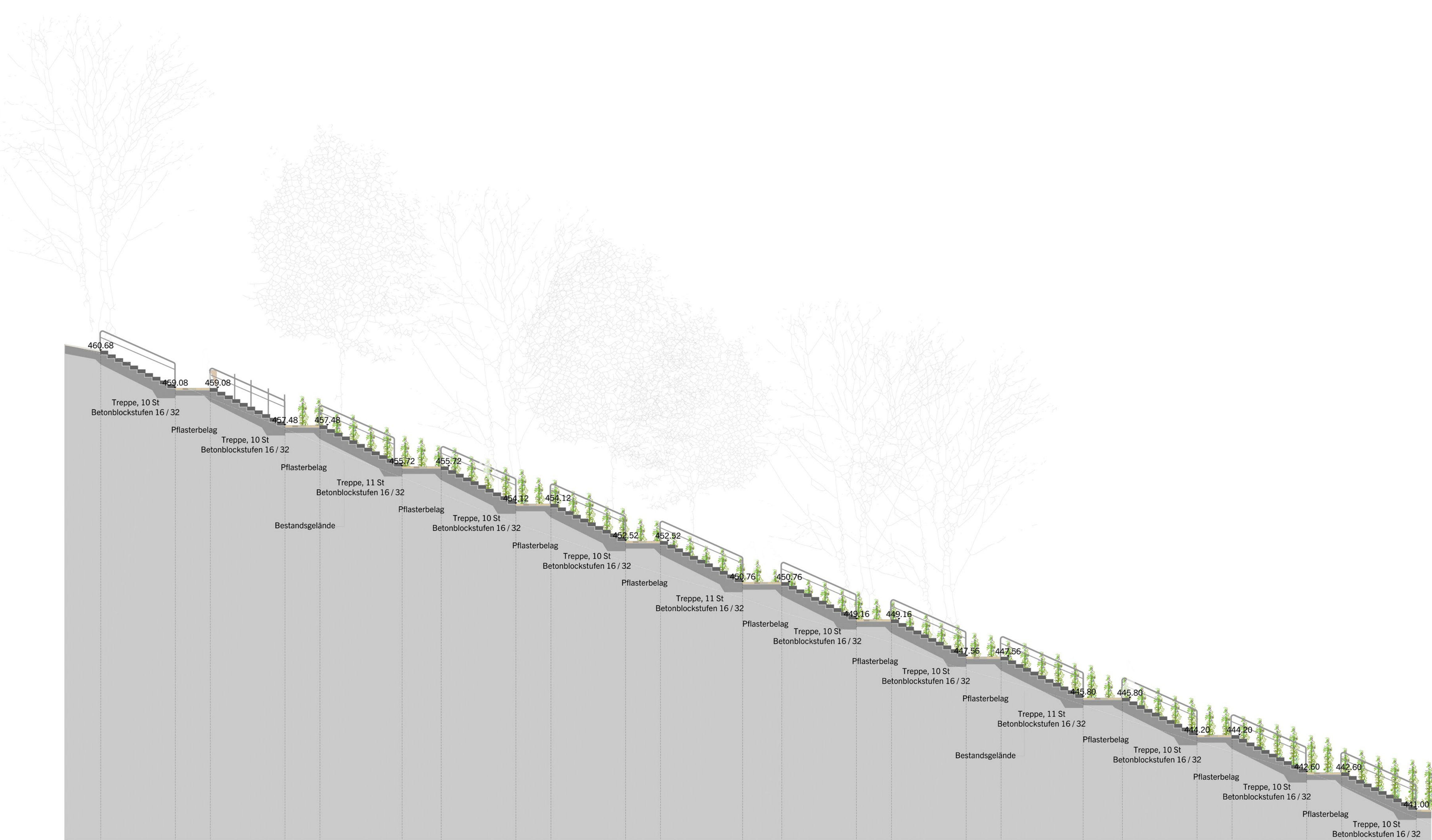
Schnitt a-a'
